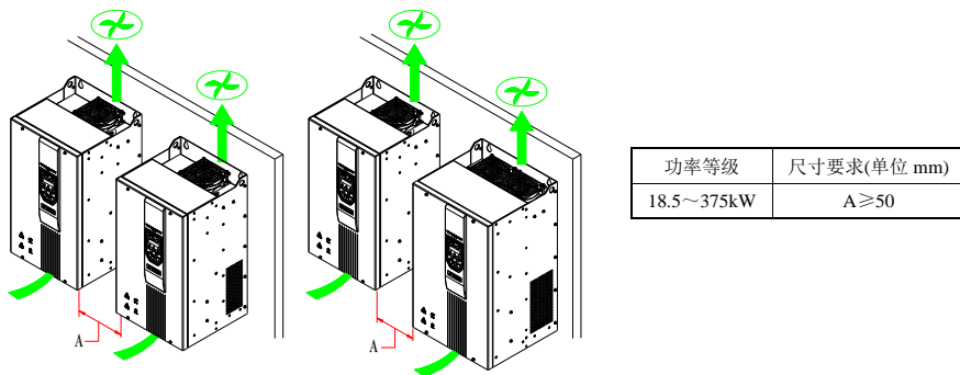
图 3-3 Hope530G18.5T6~Hope530G375T6 多台机器并排安装
