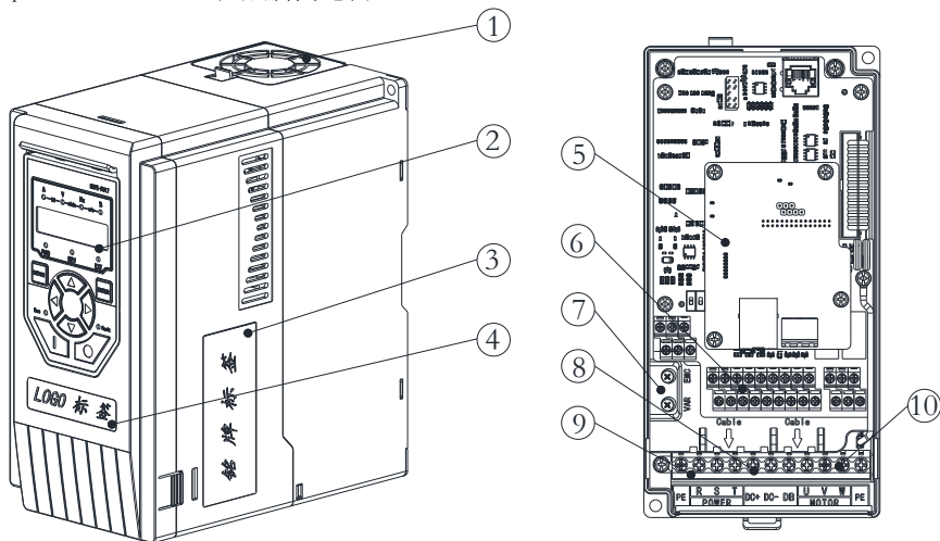
Hope500PM0.75T4~4T4 -产品部件示意图
