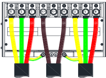
主回路端子整体接线效果图
