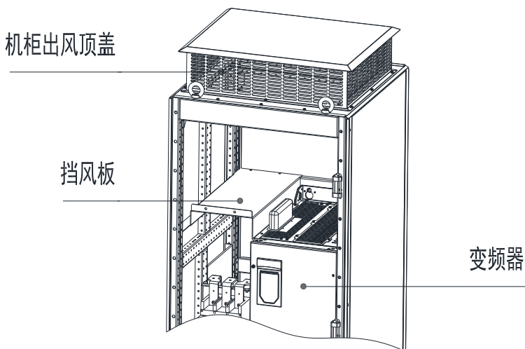
图 3-15 机柜挡风板示意图
