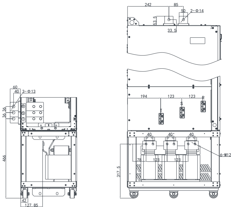
Hope500PM355~400T4L2 机型主回路端子尺寸（带输出电抗器）（mm）
