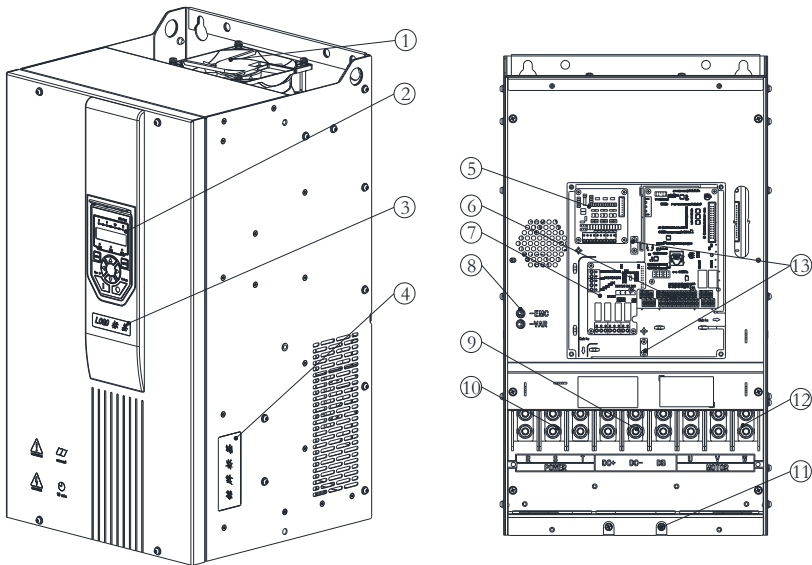
Hope500PM45T4~55T4-产品部件示意图
