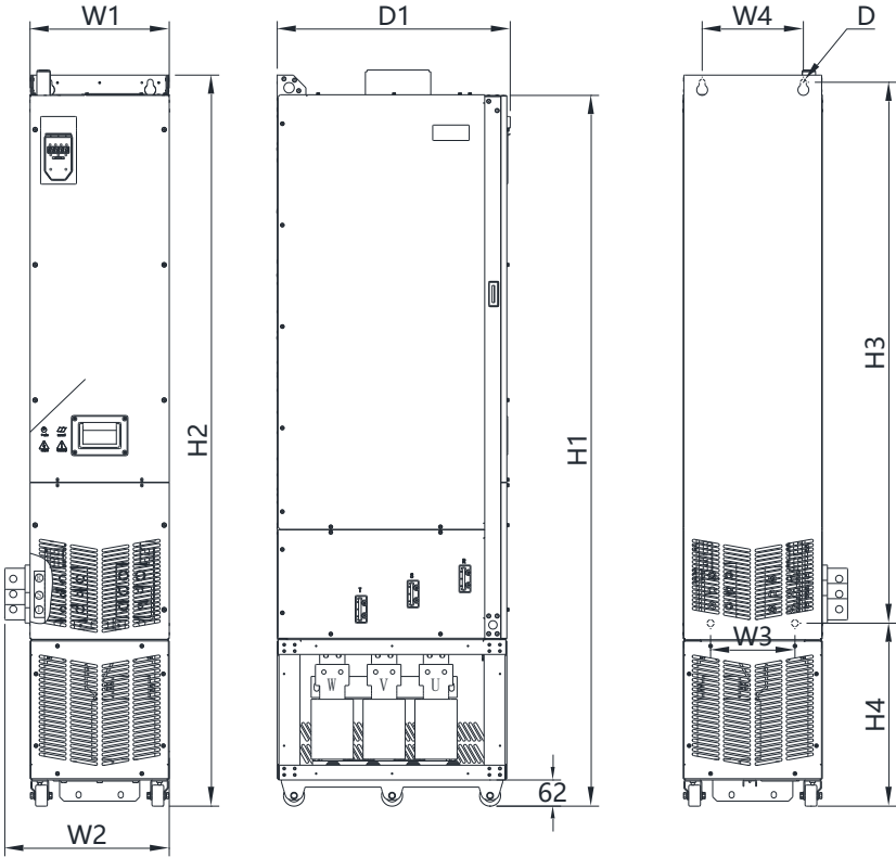
Hope500PM200~400T4L2 外形尺寸及安装尺寸示意图（含交流输出电抗器）
