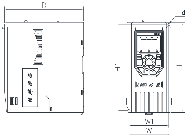
2) Hope500PM5.5T4~Hope500PM7.5T4机型安装尺寸、重量及外形图:
