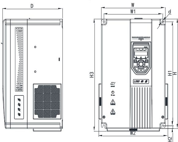
带防护罩
