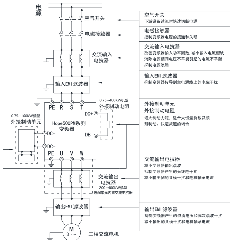
图3-14 Hope500PM系列变频系统连接示意图
