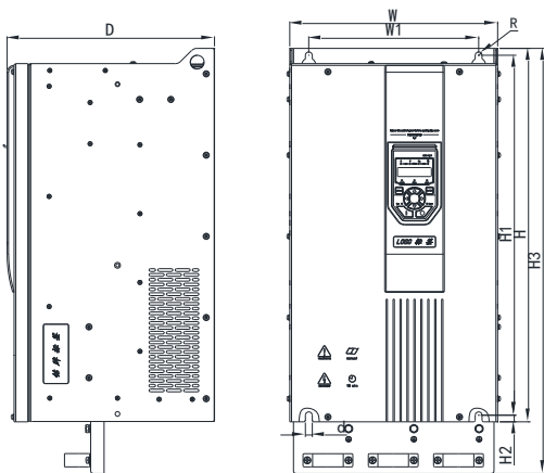
带线缆支架
