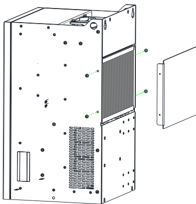
图3-14 Hope500PM底部散热器清灰示意图（45kW~160kW）
