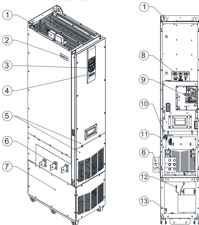
Hope500PM250T4L2~315T4L2 -产品部件示意图
