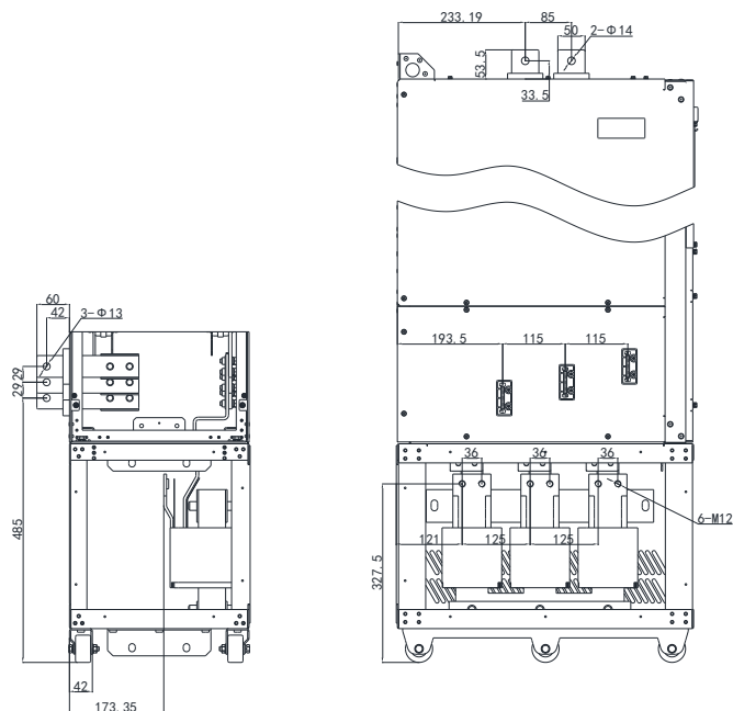
Hope500PM200~220T4L2 机型主回路端子尺寸（带输出电抗器）（mm）
