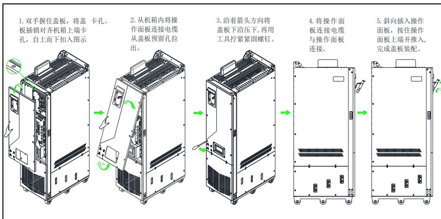
图 3-25 Hope500PM200T4~Hope500PM400T4L 机型盖板拆卸与安装步骤
