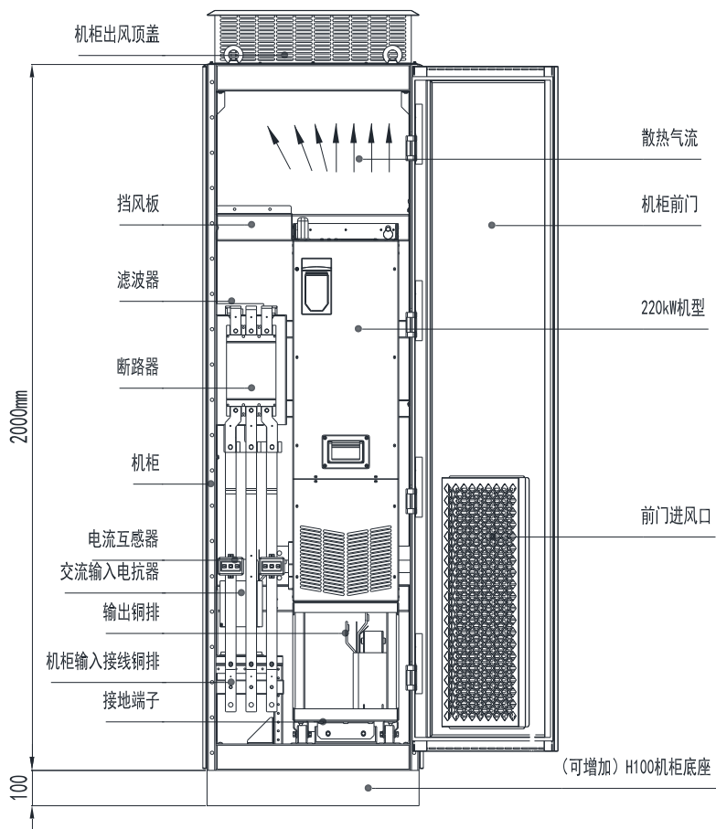
图 3-16 200kW 机型机柜布局推荐
