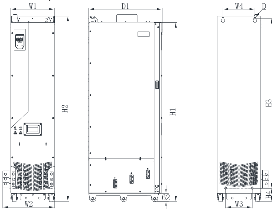
Hope500PM200~400T4L 外形尺寸及安装尺寸示意图（不含交流输出电抗器）
