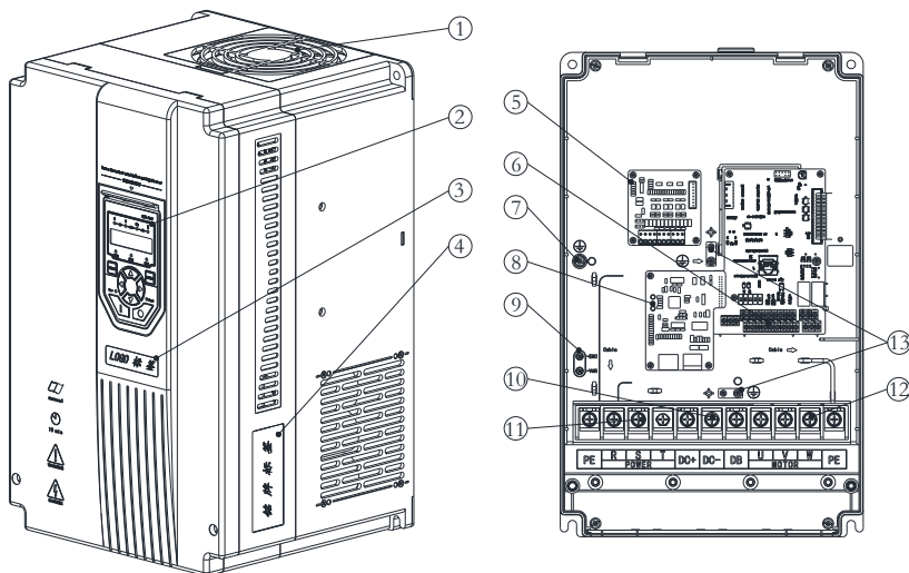
Hope500PM30T4~37T4-产品部件示意图
