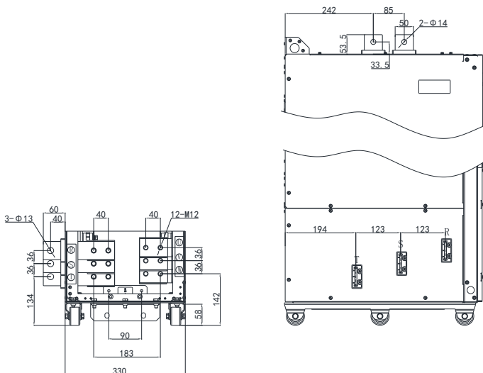
Hope500PM355~400T4L2 机型主回路端子尺寸（带输出电抗器）（mm）
