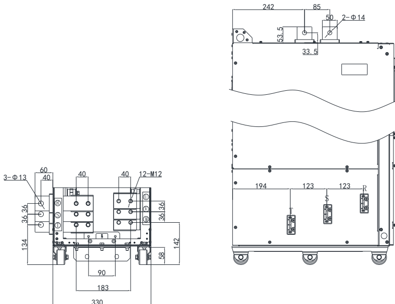
Hope500PM250~315T4L 机型主回路端子尺寸 (不带输出电抗器) (mm)
