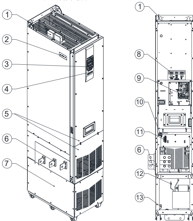
Hope500PM200T4L2~220T4L2 -产品部件示意图
