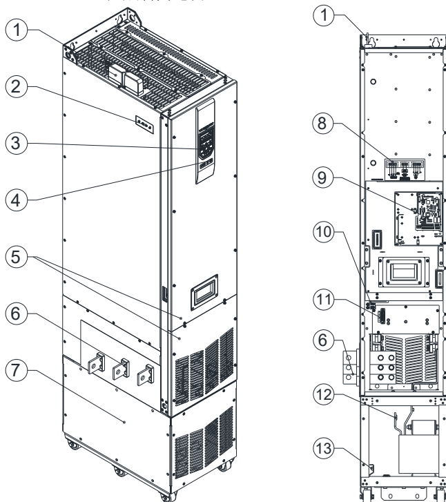
Hope500PM355T4L2~400T4L2 -产品部件示意图
