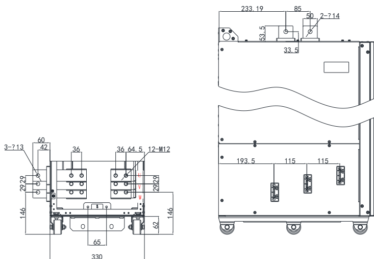
Hope500PM200~220T4L2 机型主回路端子尺寸（带输出电抗器）（mm）
