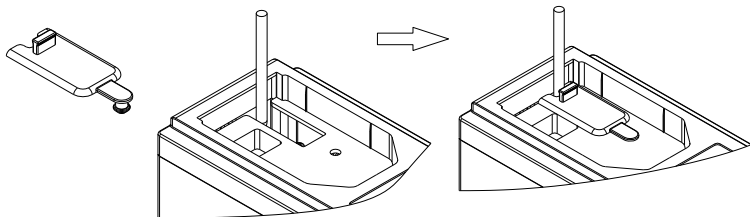
图3-13 Hope500PM0.75-7.5T4B(L)操作面板外引时橡胶塞装配示意图
