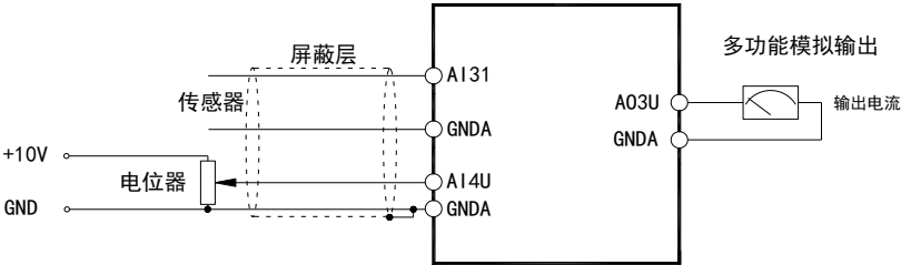
SL510-AIO1、SL530-AIO1接线示意图
