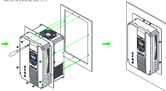
图 3-8 Hope500G11T4~Hope500G37T4 机型嵌入式安装
