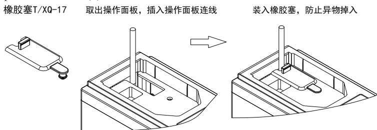
图3-13 Hope500G0.75-7.5T4B(L)操作面板外引时橡胶塞装配示意图
