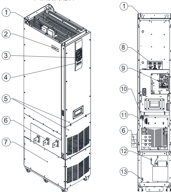
Hope500G355T4L2~400T4L2 -产品部件示意图
