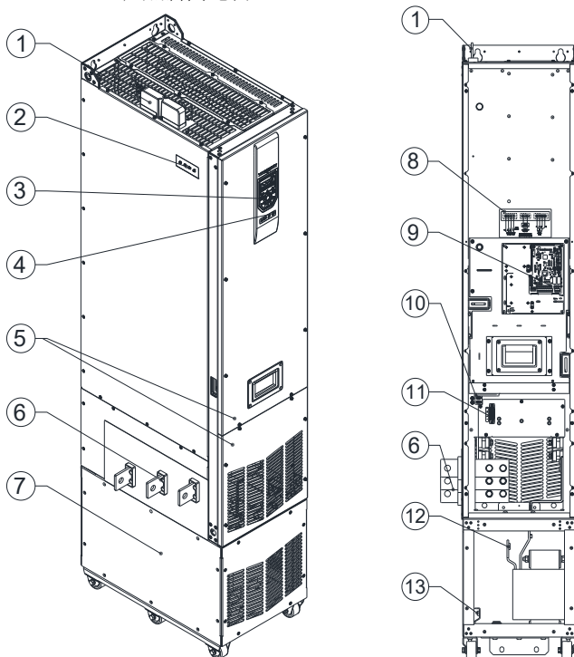
Hope500G200T4L2~220T4L2 -产品部件示意图
