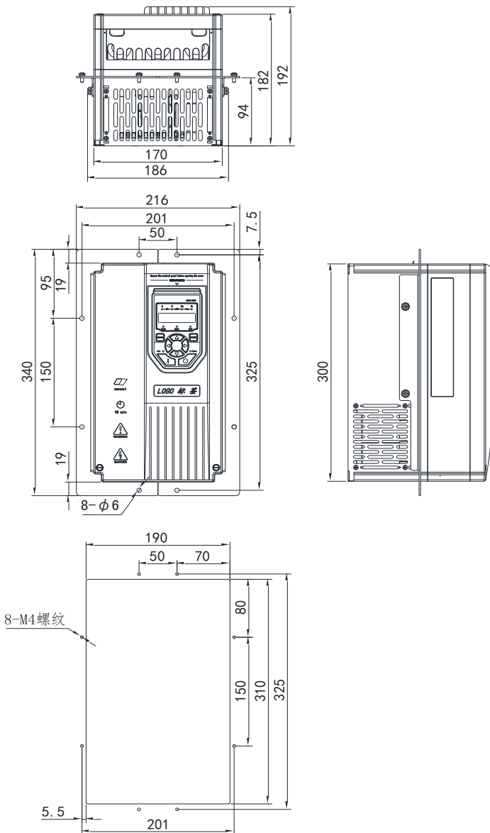
H510-A-1 安装挂条及开孔尺寸示意图
