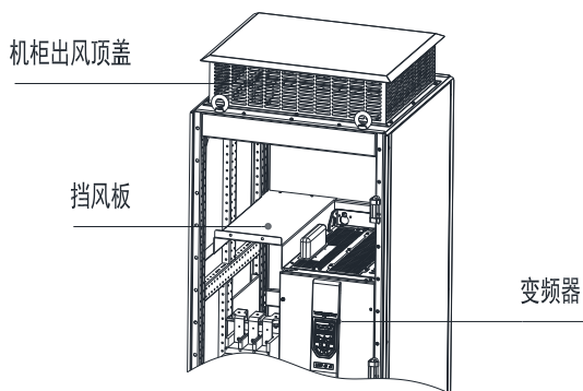
图 3-15 机柜挡风板示意图
