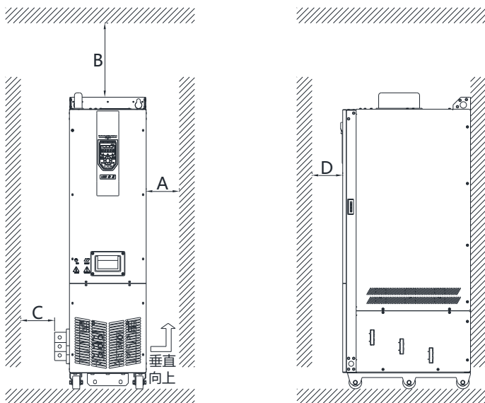
图 3-5 安装空间要求示意图
