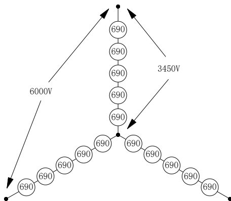
电压叠加原理图
