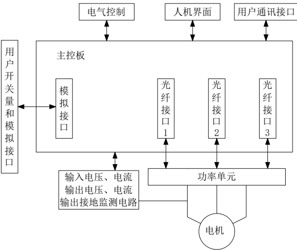
主控系统框图
