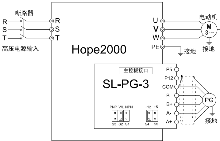
编码器接口板端子功能及规格如下表：
