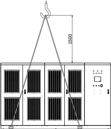
整体吊装示意图
