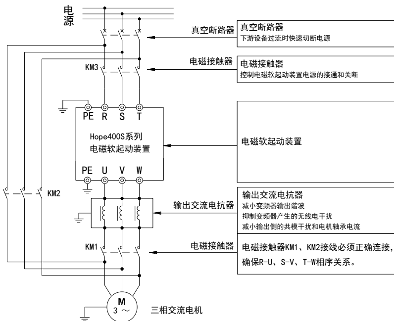
图3-9 Hope400S系列电磁软起系统连接示意图
