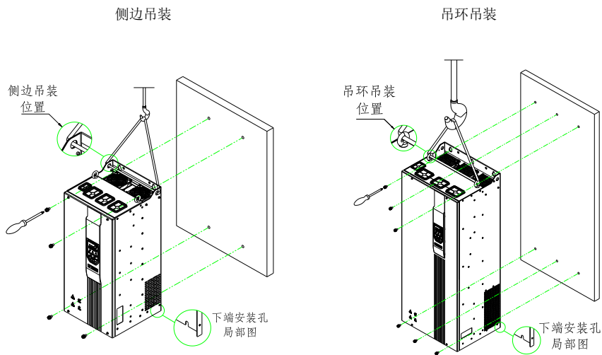
图 3-6 壁挂式安装
