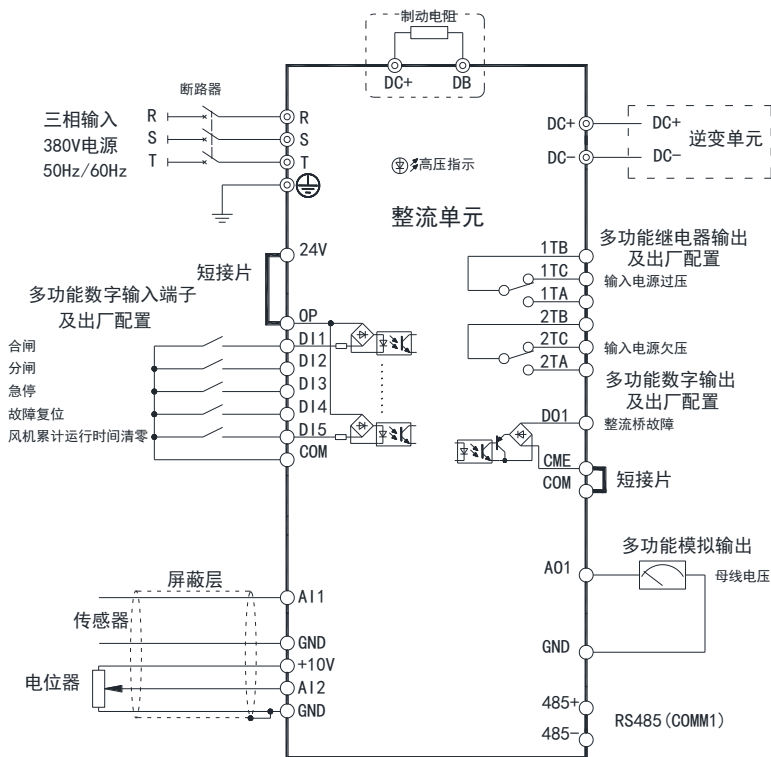
整流单元主回路端子功能说明
