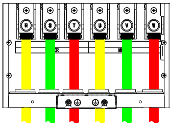
主回路输入输出端子接线效果图
