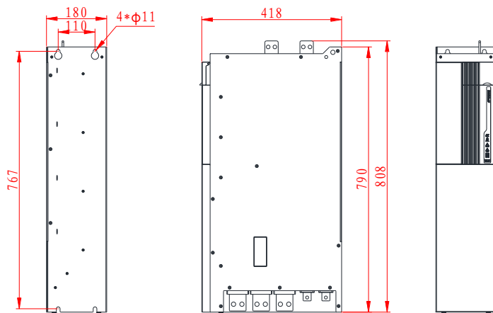
4) Hope600-M20-C0625-A4机型(整流单元)安装尺寸及外形图:
