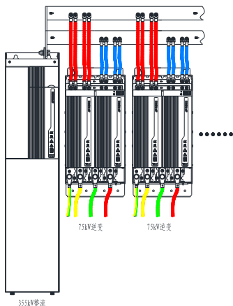
直流母线外引线缆方式整体接线示意图
