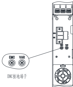
整流单元限位螺钉示意图
