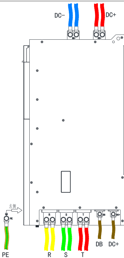
355kW 整流单元 接线示意图
