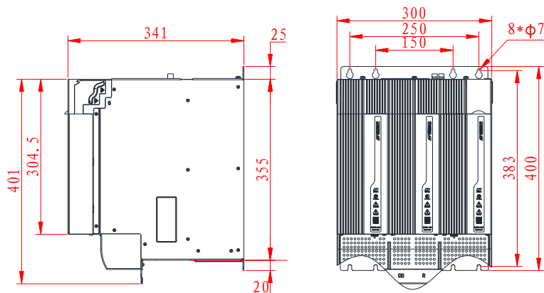
4) Hope600-M20-C0625-A4机型(整流单元)安装尺寸及外形图:
