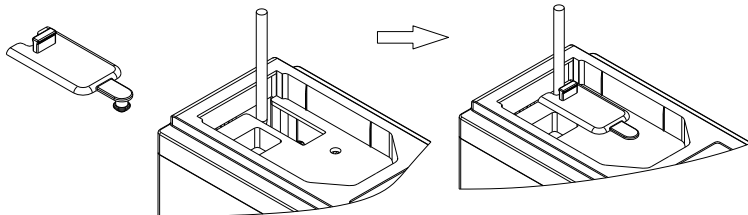
图3-13 Hope530G0.75-7.5T4B(L)操作面板外引时橡胶塞装配示意图
