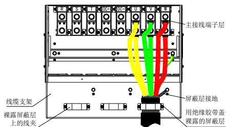
主回路端子输出端接线效果图
