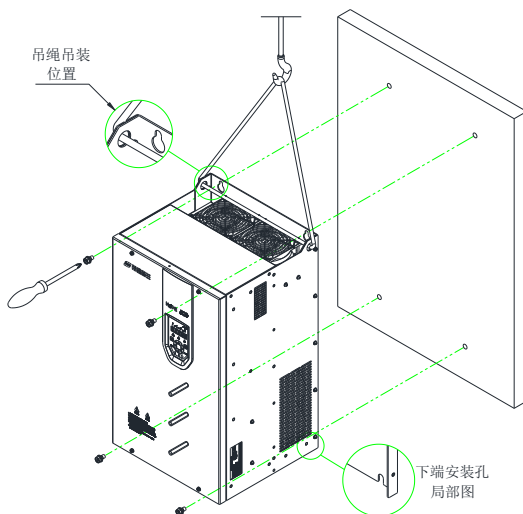
图 3-7 Hope510PM45T4~Hope510PM375T4 机型壁挂式安装
