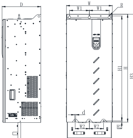
200~375kW 带线缆支架
