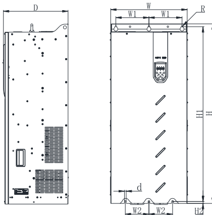
200~375kW 带线缆支架
