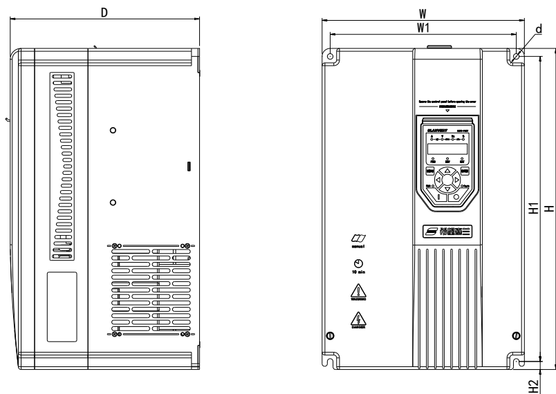
不带防护罩
