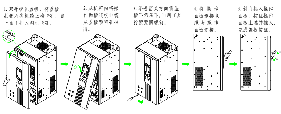
图 3-12 Hope530G45T4~Hope530G375T4 机型盖板拆卸与安装步骤
