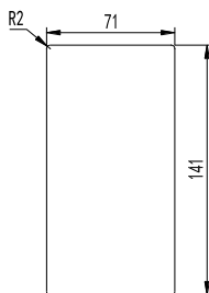
机柜开孔尺寸
