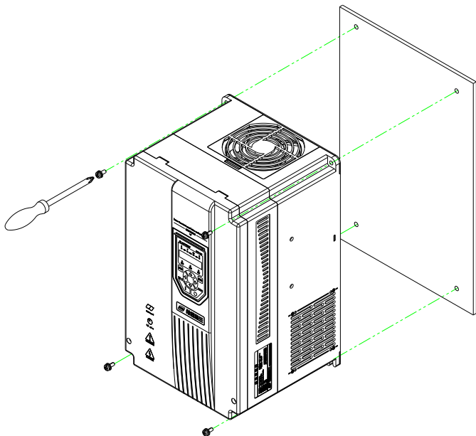
图 3-6 Hope530G0.75T4~Hope530G375T4 机型壁挂式安装
