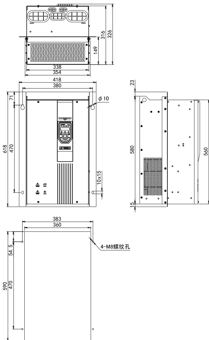
H510-A-5 安装挂条及开孔尺寸示意图
