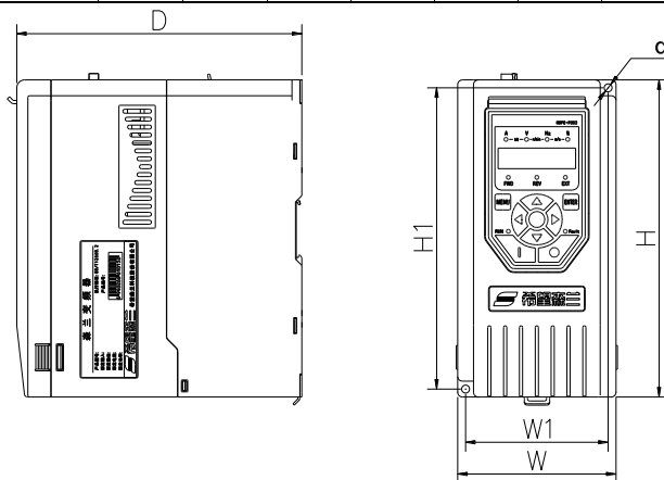
2) Hope530G5.5T4~Hope530G7.5T4机型安装尺寸、重量及外形图:
