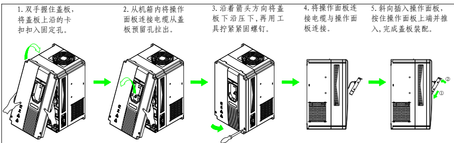
图 3-11 Hope530G11T4~Hope530G37T4 机型盖板拆卸与安装步骤
