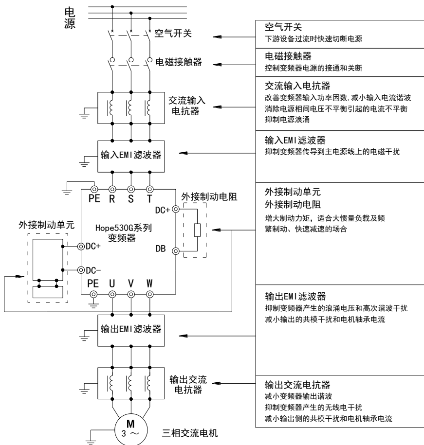
图3-13 Hope530系列变频系统连接示意图
