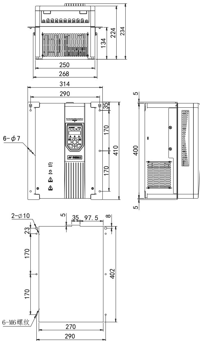
H510-A-3 安裝挂條及開孔尺寸示意圖
