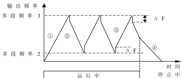
图 6-26 摆频运行
