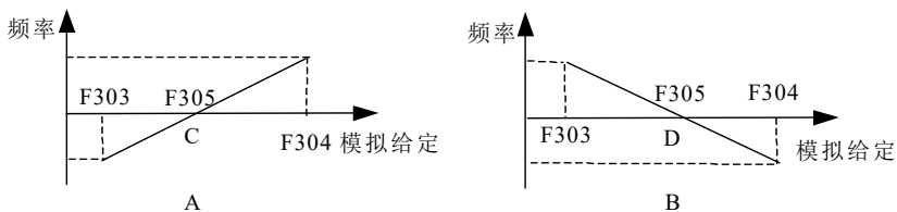
图 6-2 模拟信号辅助给定
