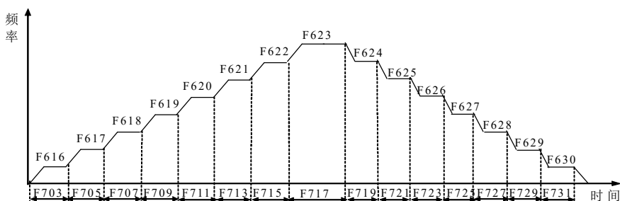
图 6-25 程序运行
