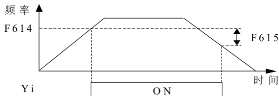
图 6-24 检出频率
