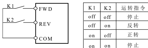
图 6-3A 两线控制模式 1
