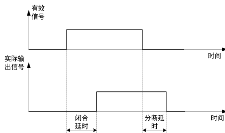
图 6-19 端子输出信号延时功能
