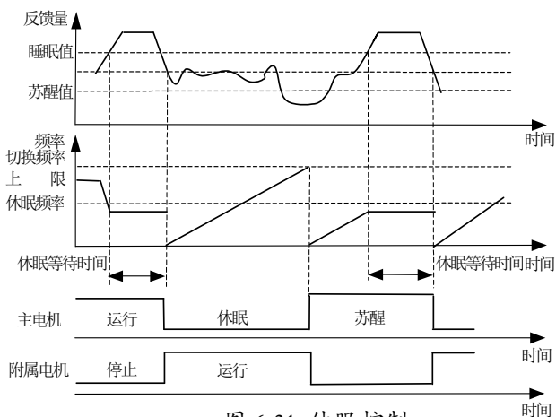
图 6-31 休眠控制
