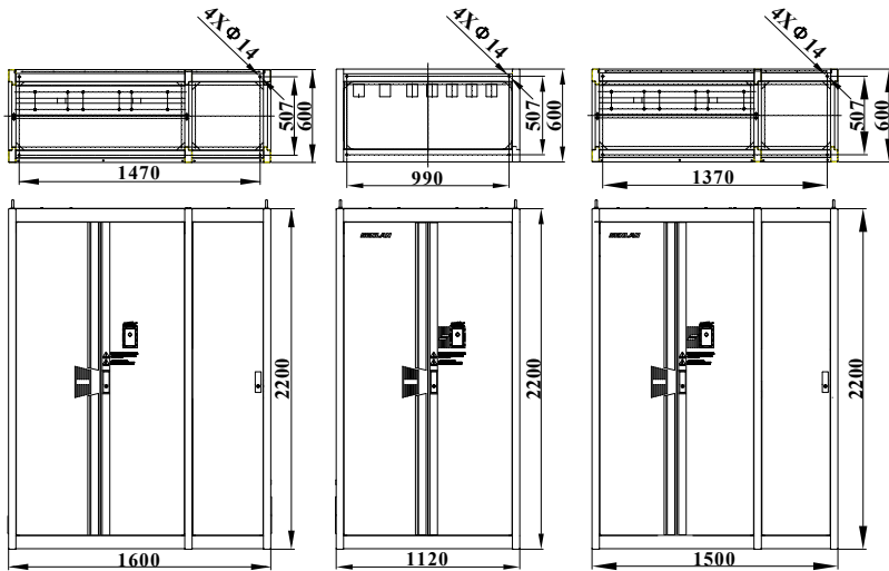
SB61G + 560C外形尺寸
