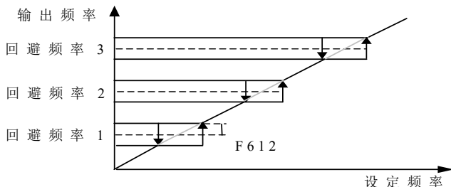
图 6-22 回避频率
