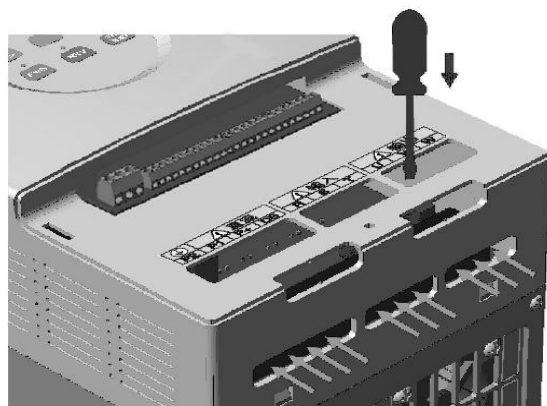
主电路接线
