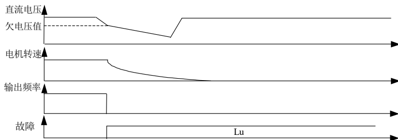
图 6-11A 再启动不动作
