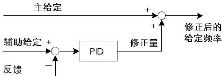
图 6-28 辅助通道 PID 调节
