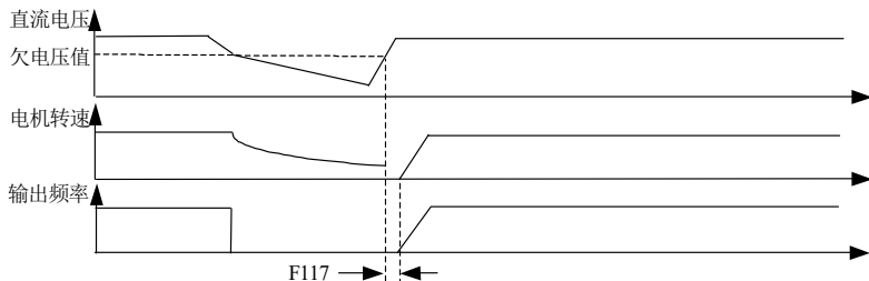
图 6-11B 频率从零再起
