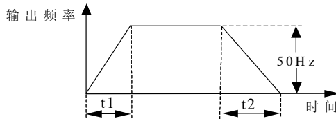
图 6-5 加、减速时间
