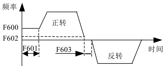
图 6-20 正反转死区时间
