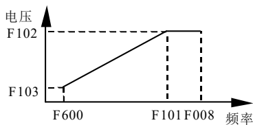
图 6-8 转矩提升
