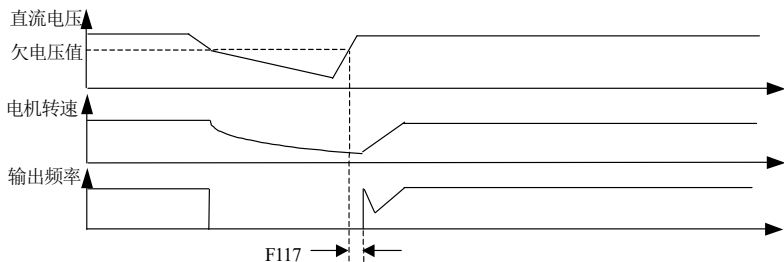
图 6-11C 转速跟踪再起
