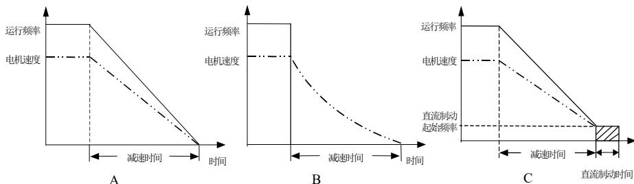
图 6-4 电机停车方式
