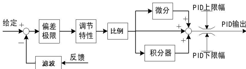
图 6-27 过程 PID
