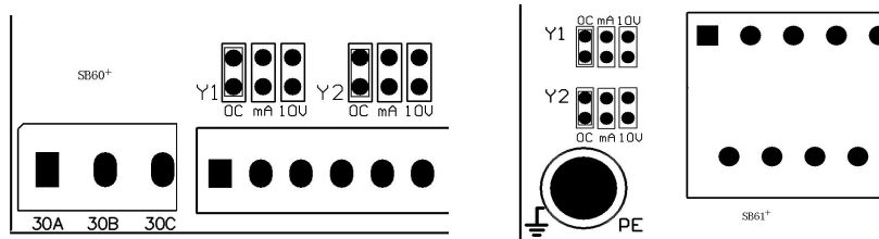
图 6-17(a) SB60 + /61 + 的 Y1、Y2 端子功能选择跳针
