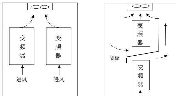
(a) 多台变频器横配置
