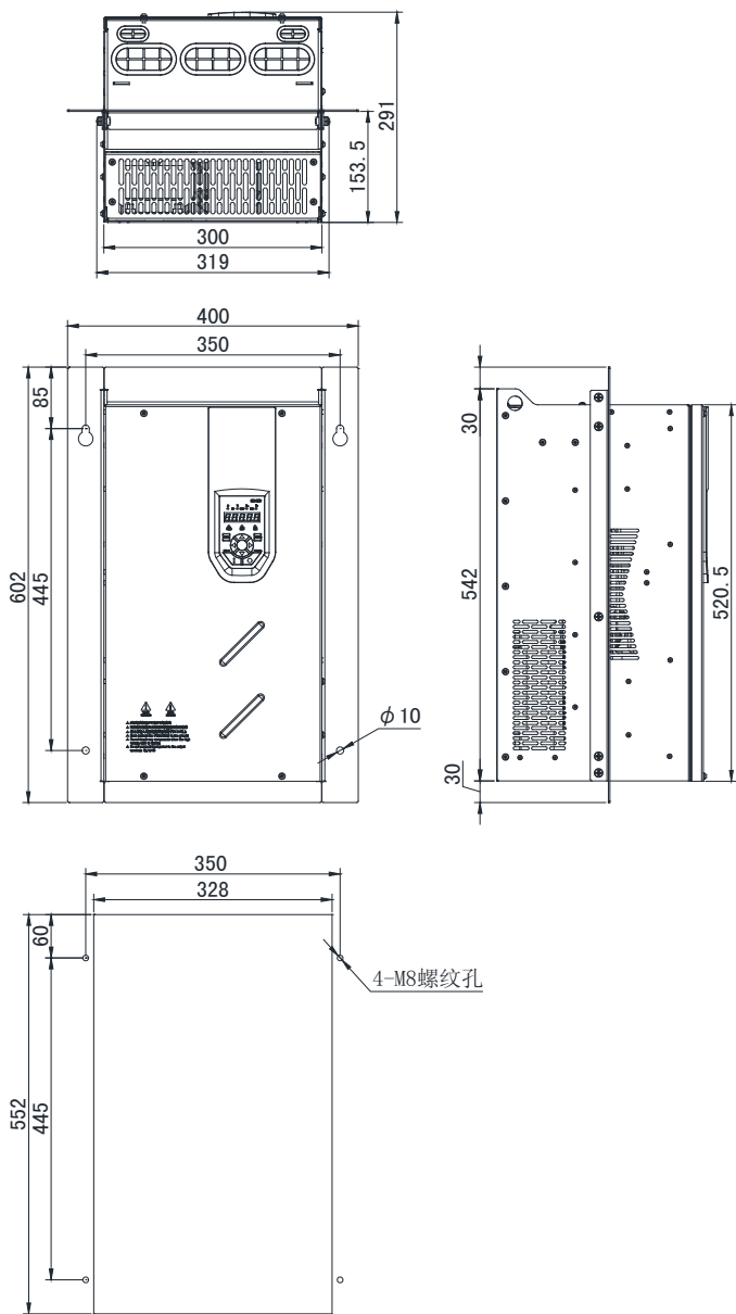
H510G-4 安装支架及开孔尺寸展示图
