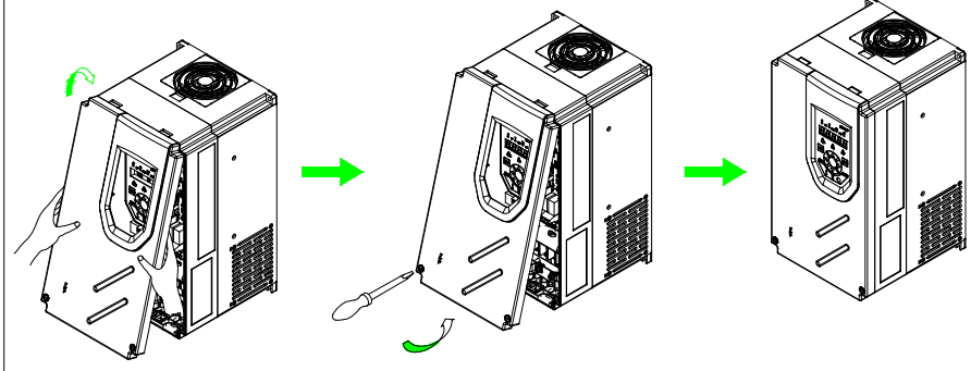
图 3-10 HOPE510G11T4~HOPE510G37T4 机型盖板拆卸与安装步骤
