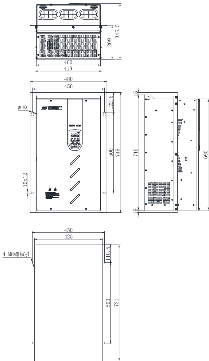
H510G-6 安装支架及开孔尺寸展示图
