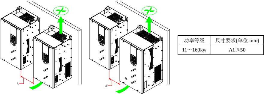
图 3-3 HOPE510G11T4~HOPE510G160T4 多台机器并排安装
