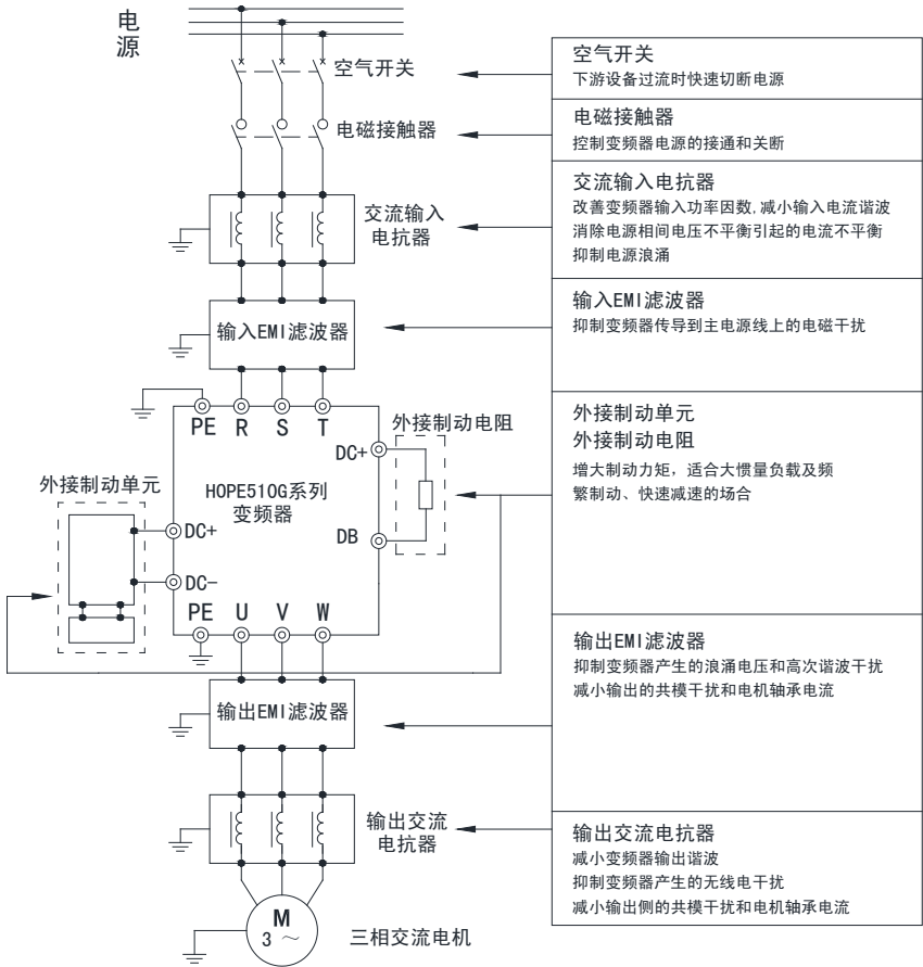
图3-12 HOPE510系列变频系统连接示意图
