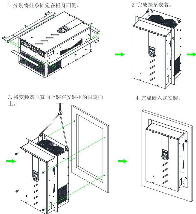
图 3-9 HOPE510G45T4~HOPE510G160T4 机型嵌入式安装
