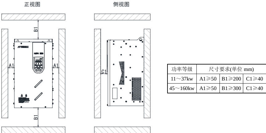
图 3-2 单台机器(HOPE510G11T4~HOPE510G160T4)安装间隔
