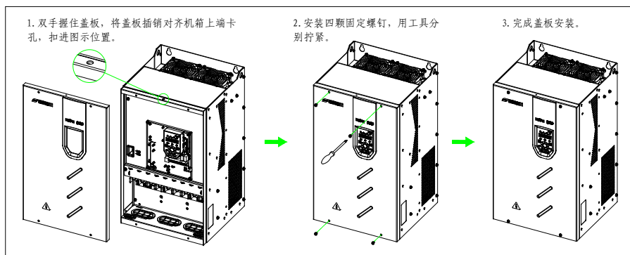
图 3-11 HOPE510G45T4~HOPE510G160T4 机型盖板拆卸与安装步骤
