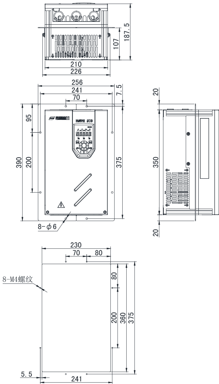
H510G-2 安装支架及开孔尺寸展示图
