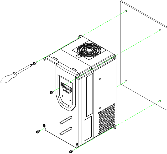
图 3-6 HOPE510G11T4~HOPE510G37T4 机型壁挂式安装
