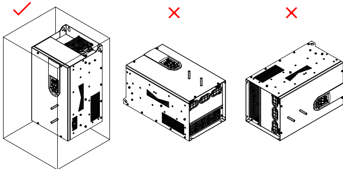
图 3-5 安装方向示意图
