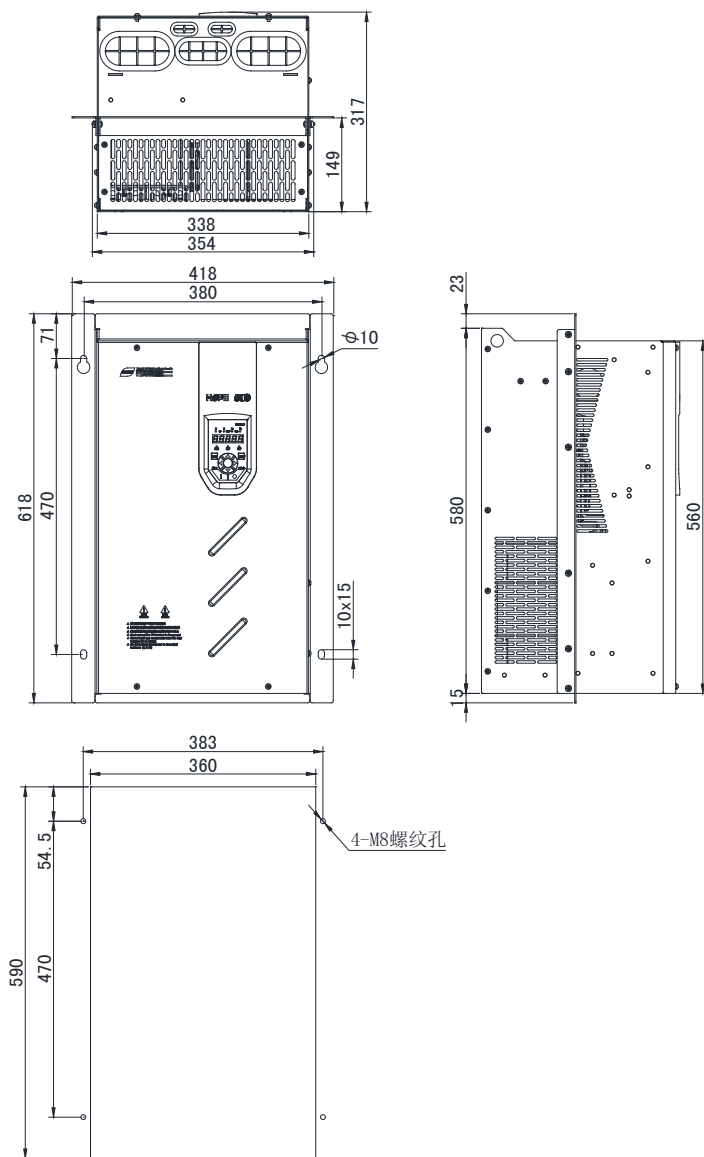
H510G-5 安装支架及开孔尺寸展示图
