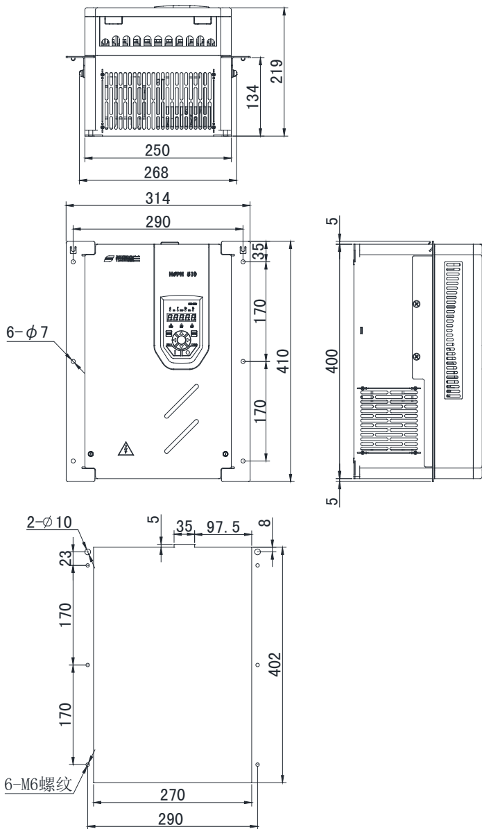
H510G-3 安装支架及开孔尺寸展示图
