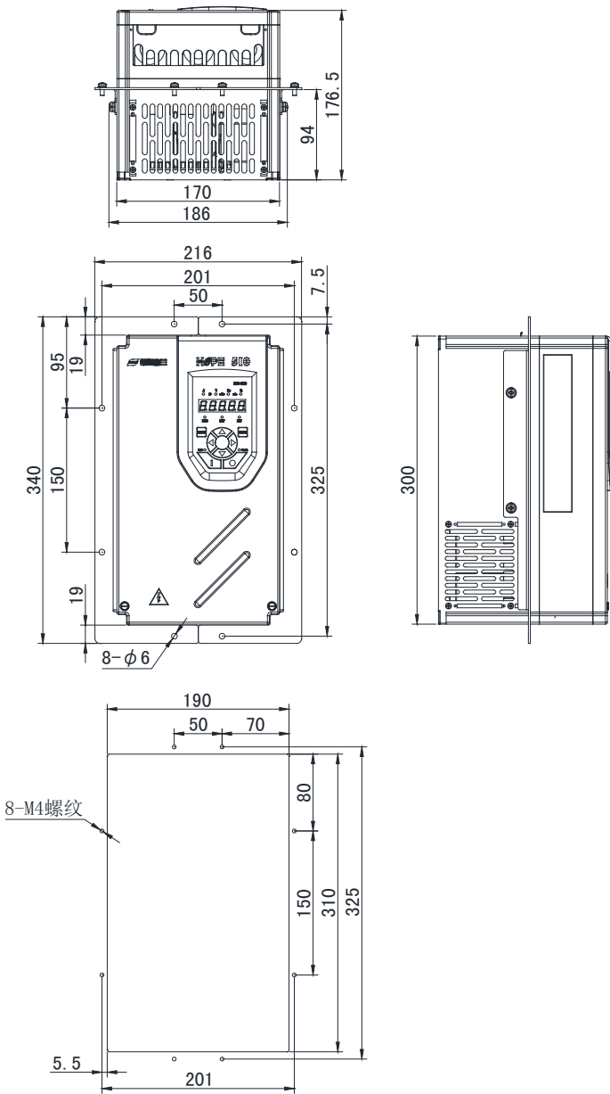
H510G-1 安装支架及开孔尺寸展示图
