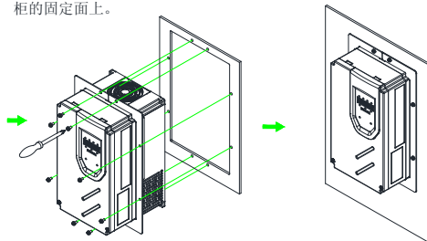
图 3-8 HOPE510G11T4~HOPE510G37T4 机型嵌入式安装
