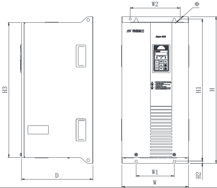
Hope800G18.5~375T4外形尺寸图:
