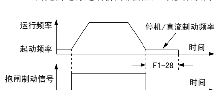
抱闸延迟时序图
