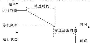
零速延迟时序图
