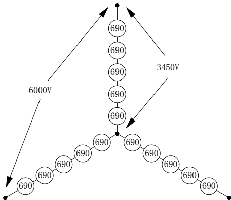
电压叠加原理图
